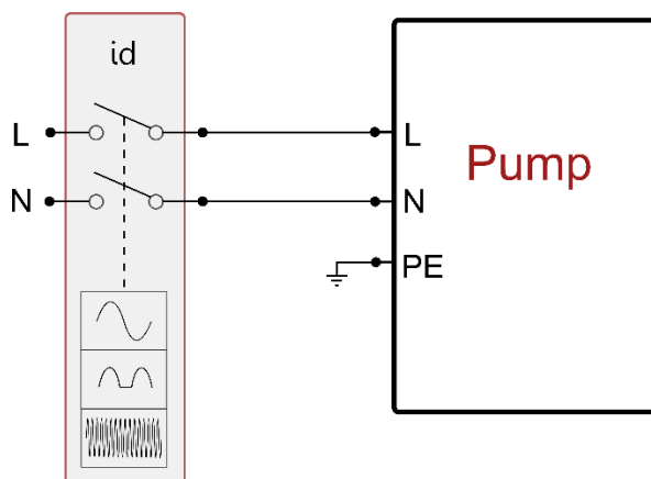
Przykład instalacji
